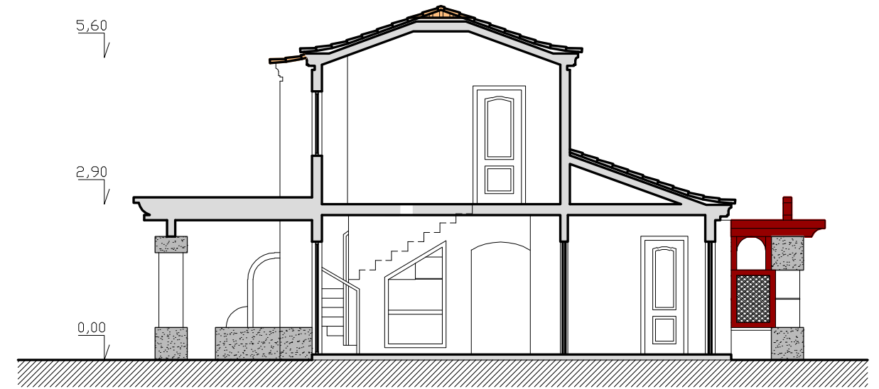
CORTE AB
